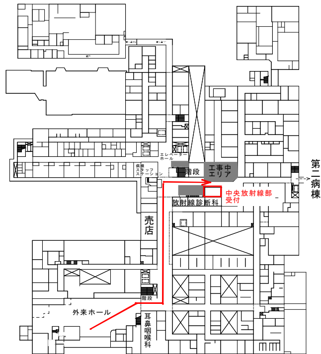
1階平面図
